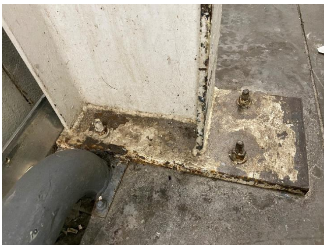
“PLACAS BASE, EN LAS COLUMNAS DE SOPORTE DE RACK DE REFRIGERACIÓN”.
